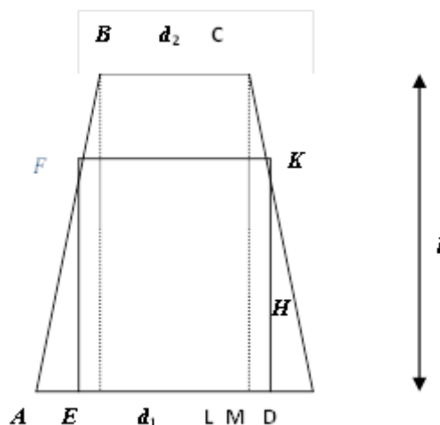
Figura 3. - Sección transversal de la troza y el prisma de mayor volumen posible a extraer de la misma
