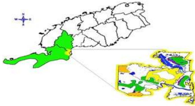
Fig. 1. Ubicación geográfica del área de estudio. Fuente: Elaboración propia.
